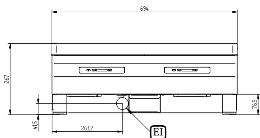
Oldalnézet
